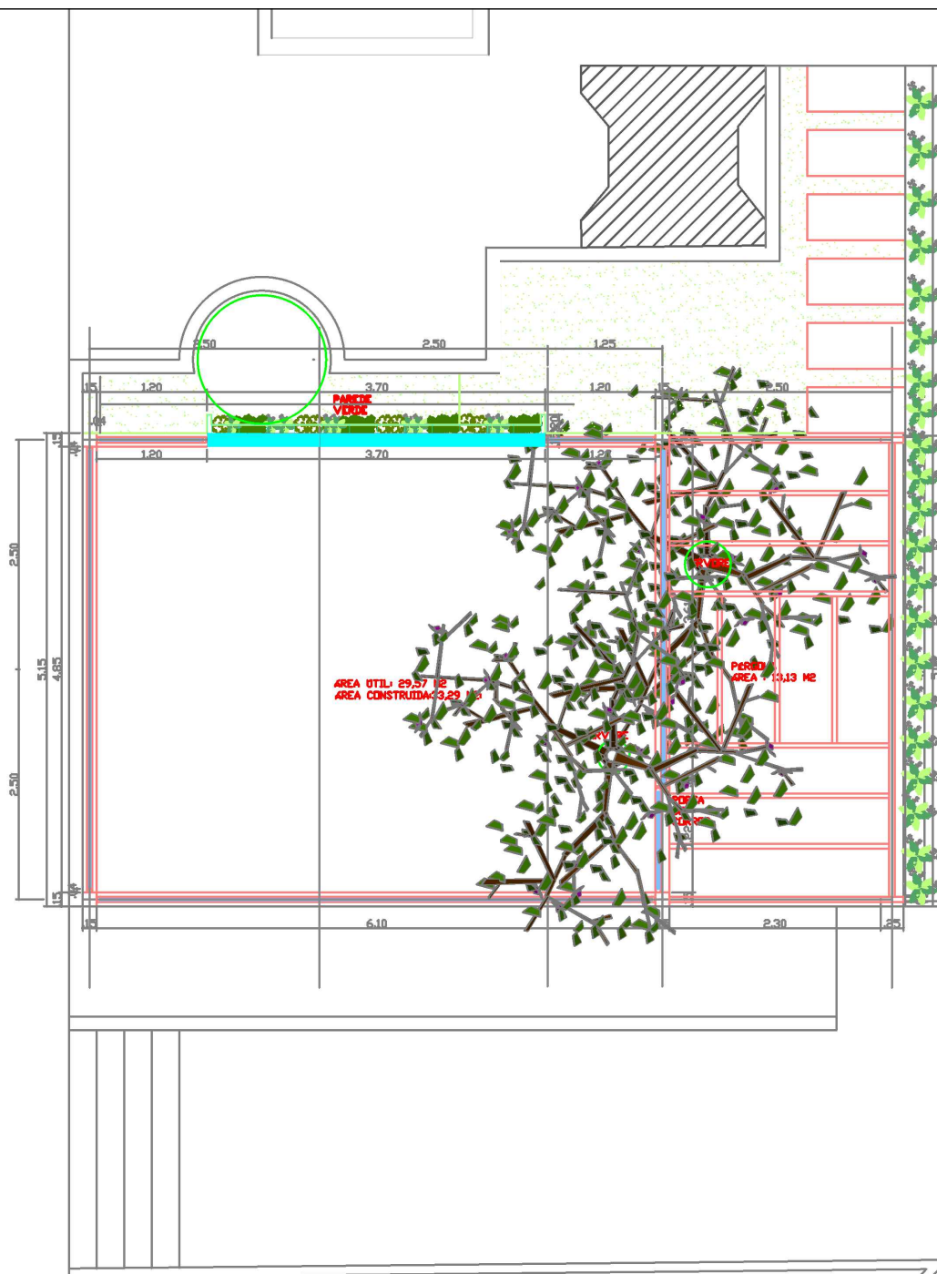
IMPLANTAÇÃO ESC. 1/75
