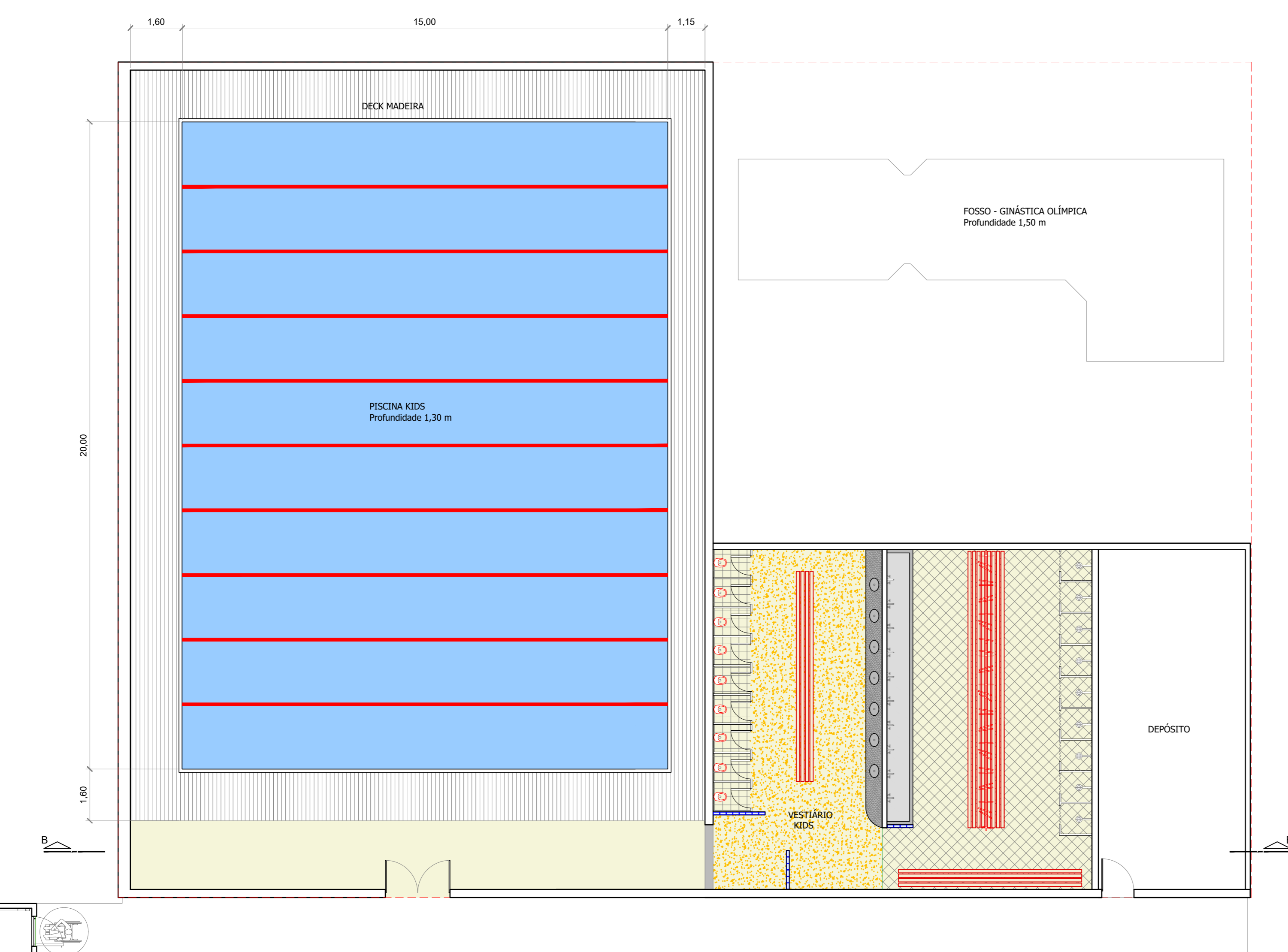
ÁREA DE AMPLIAÇÃO NÍVEL -1 ESC. 1:100
