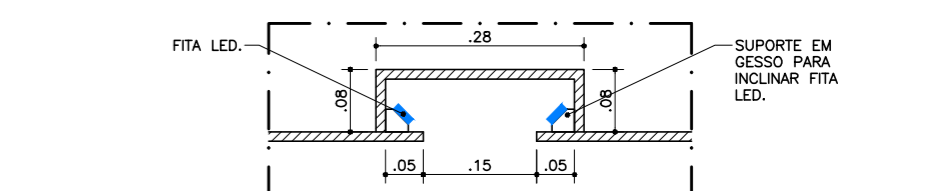
DETALHA DE SANCA 03 ESC. 1:10
