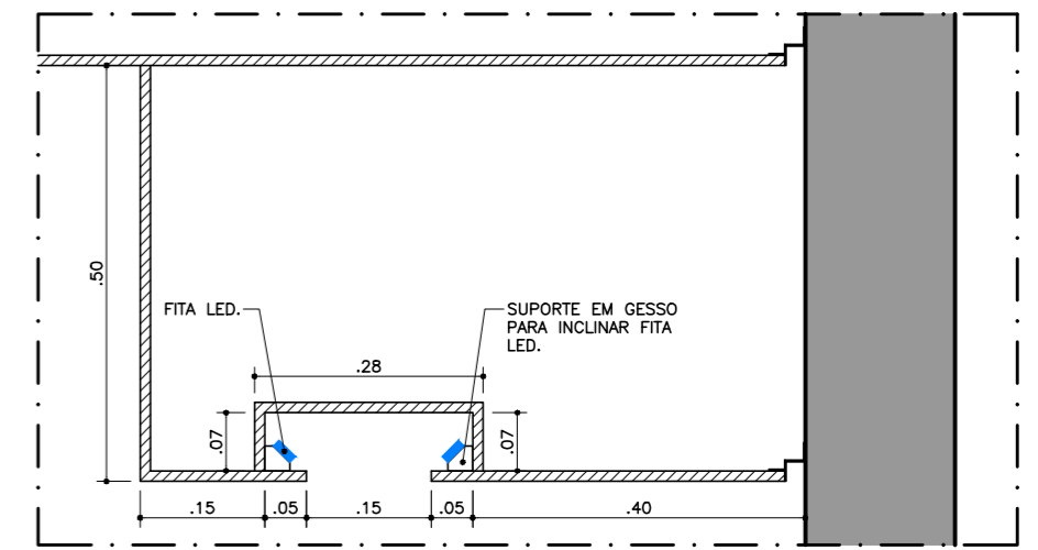
DETALHA DE SANCA 01 ESC. 1:10
