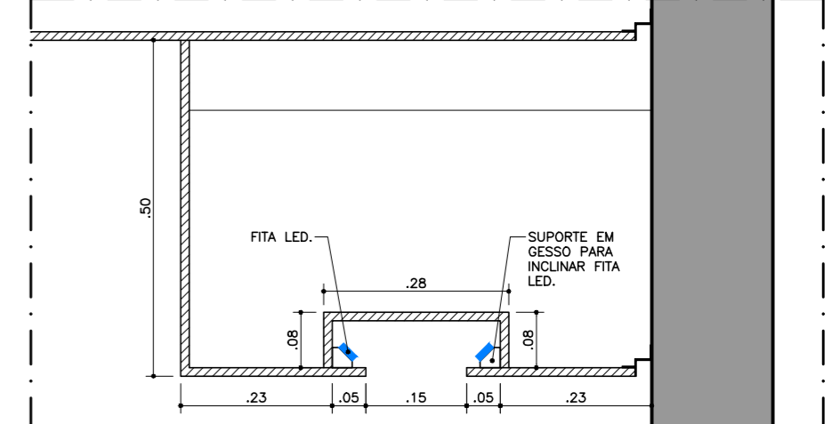
DETALHA DE SANCA 02 ESC. 1:10
