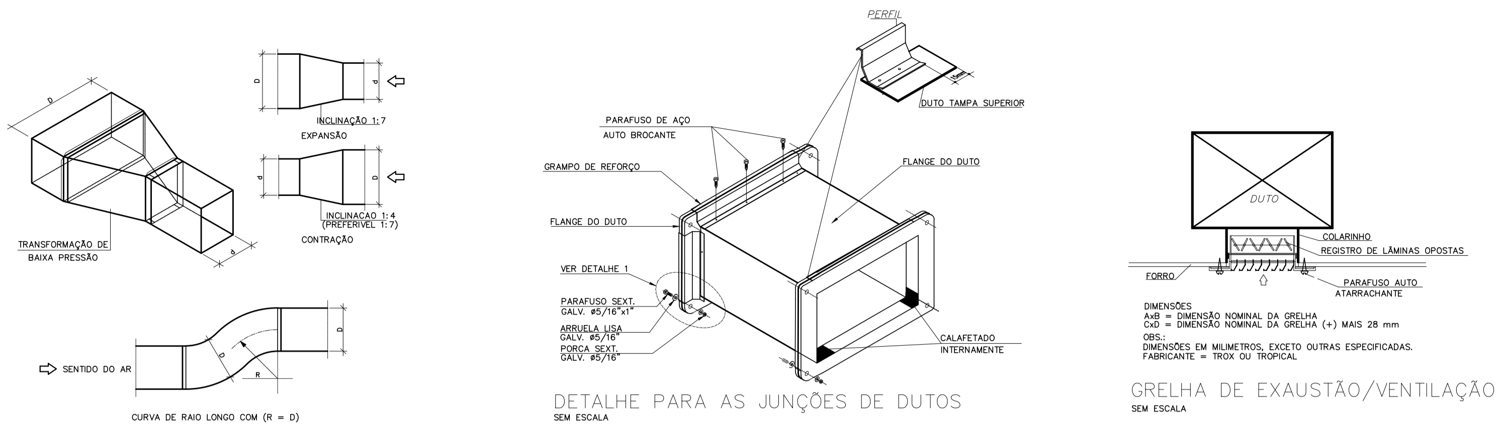
DETALHE DE CONSTRUÇÃO DAS EXPANSÕES CONTRAÇÕES DE DUTOS SEM ESCALA
