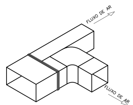
DETALHE DE CONSTRUÇÃO DE RAMIFICAÇÕES DE DUTOS SEM ESCALA
