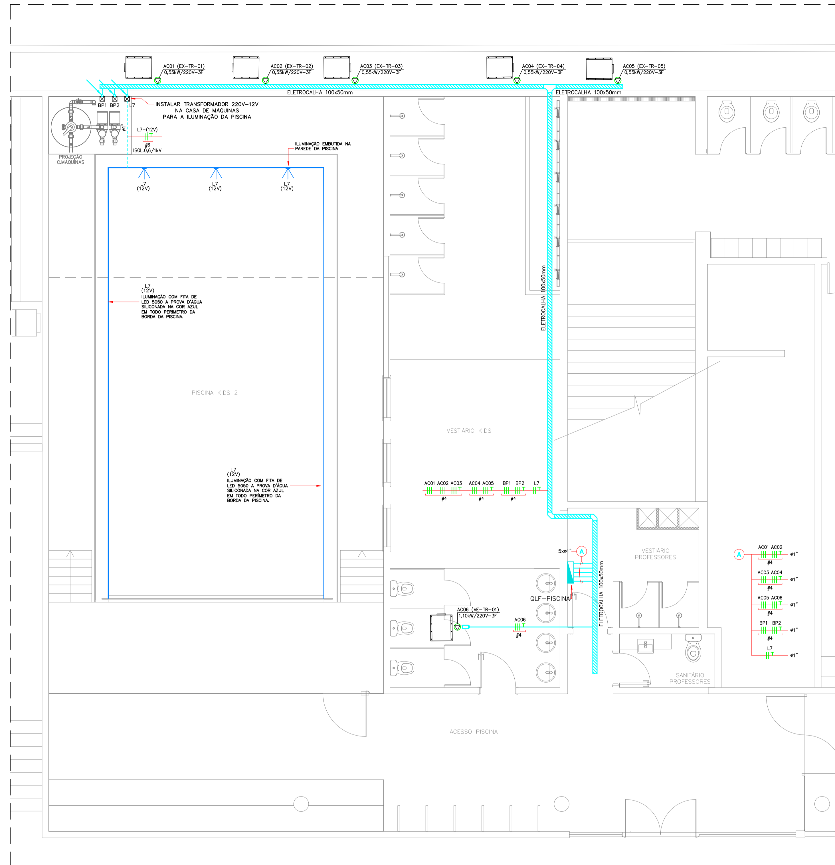
PAVIMENTO TÉRREO – PONTOS DE FORÇA / ILUM. PISCINA ESCALA 1:50
