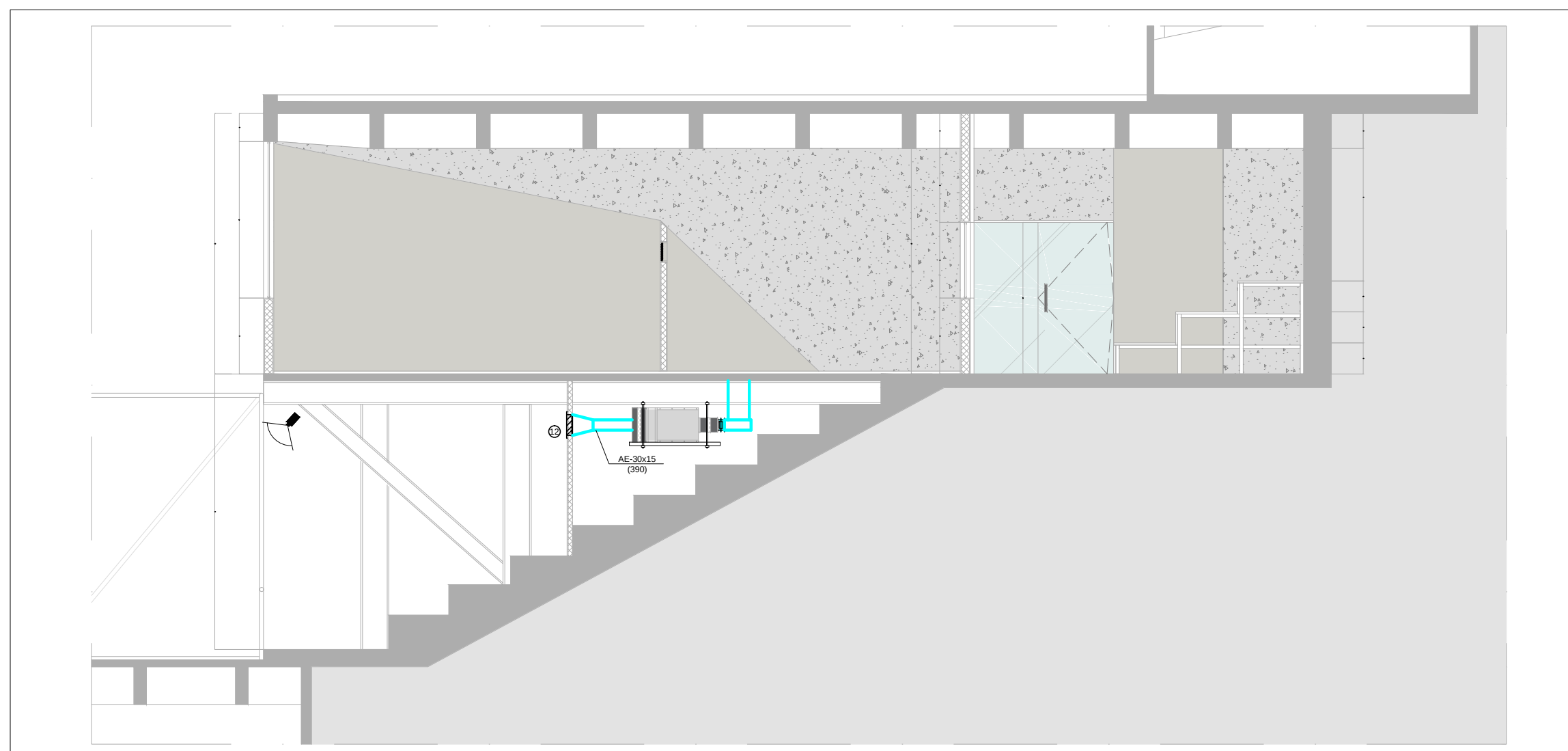
01 CORTE CC ESCALA: 1/75
