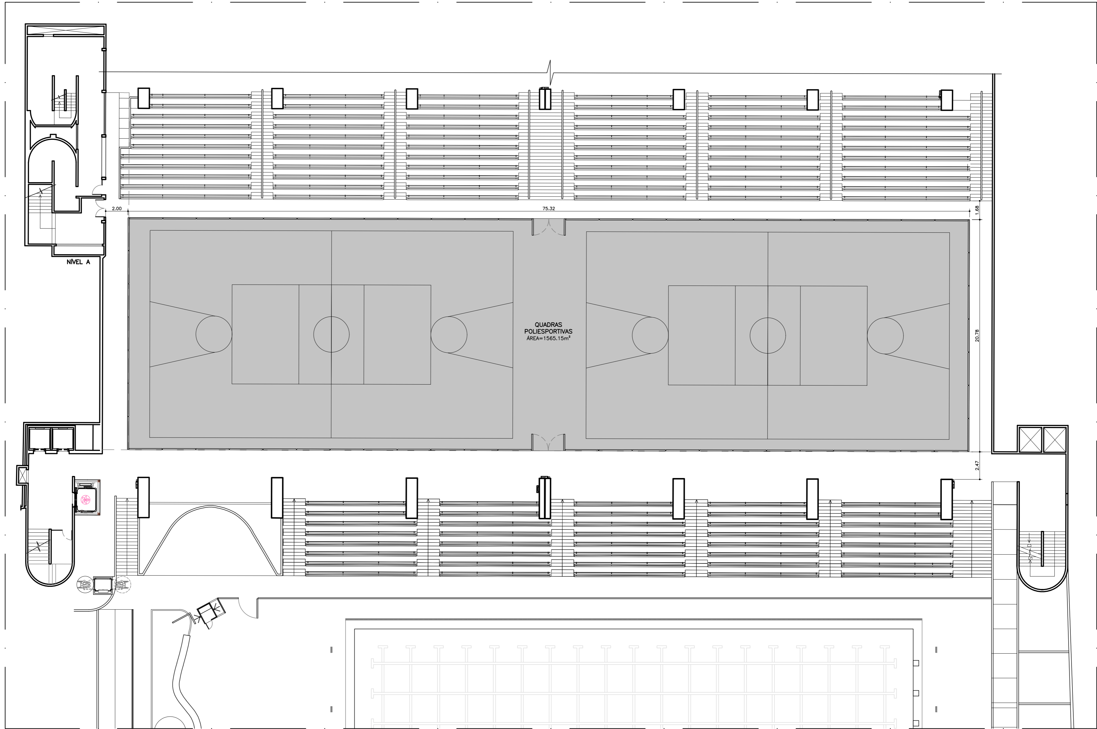
QUADRAS POLIESPORTIVAS ESC. 1:200
