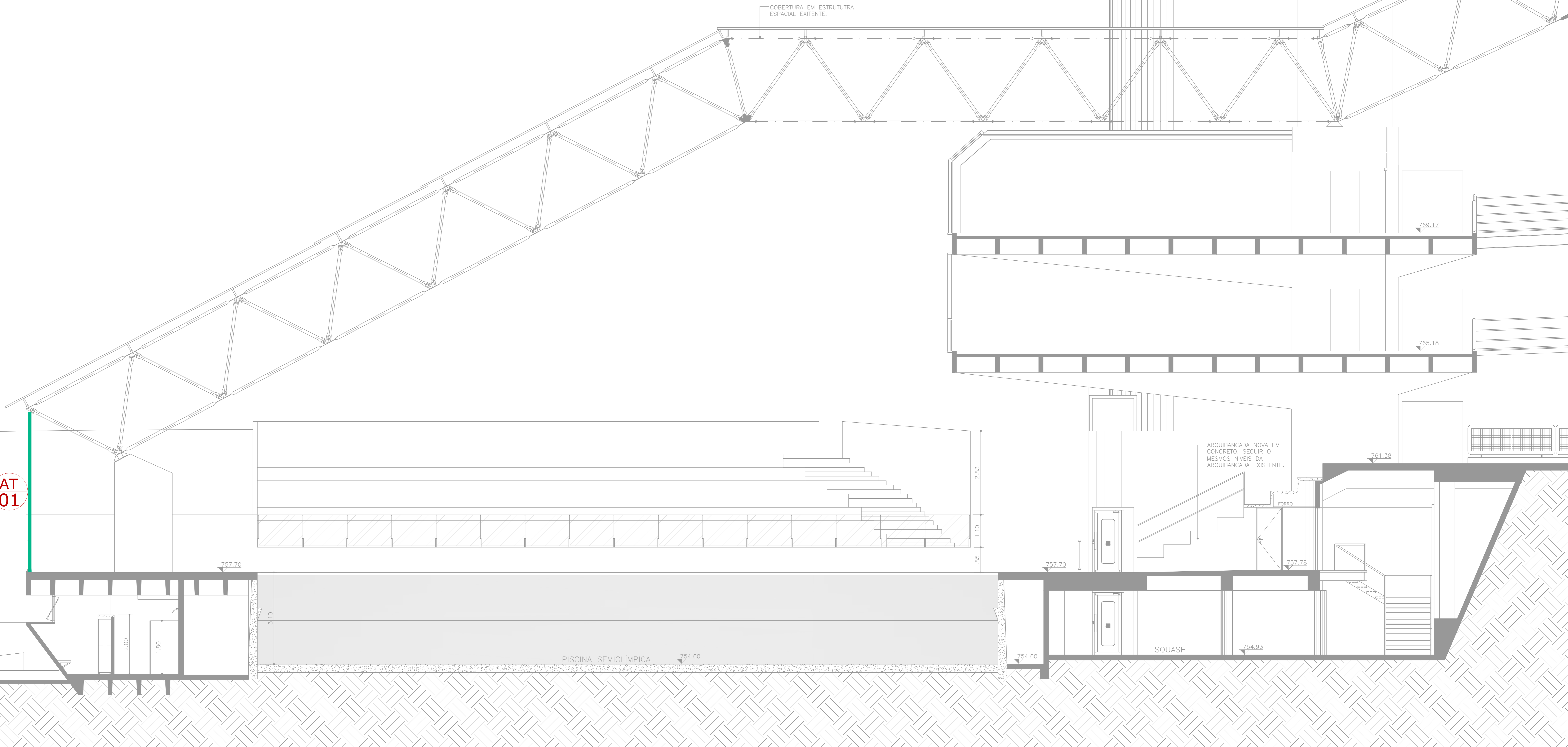
CORTE BB ESC. 1:50
