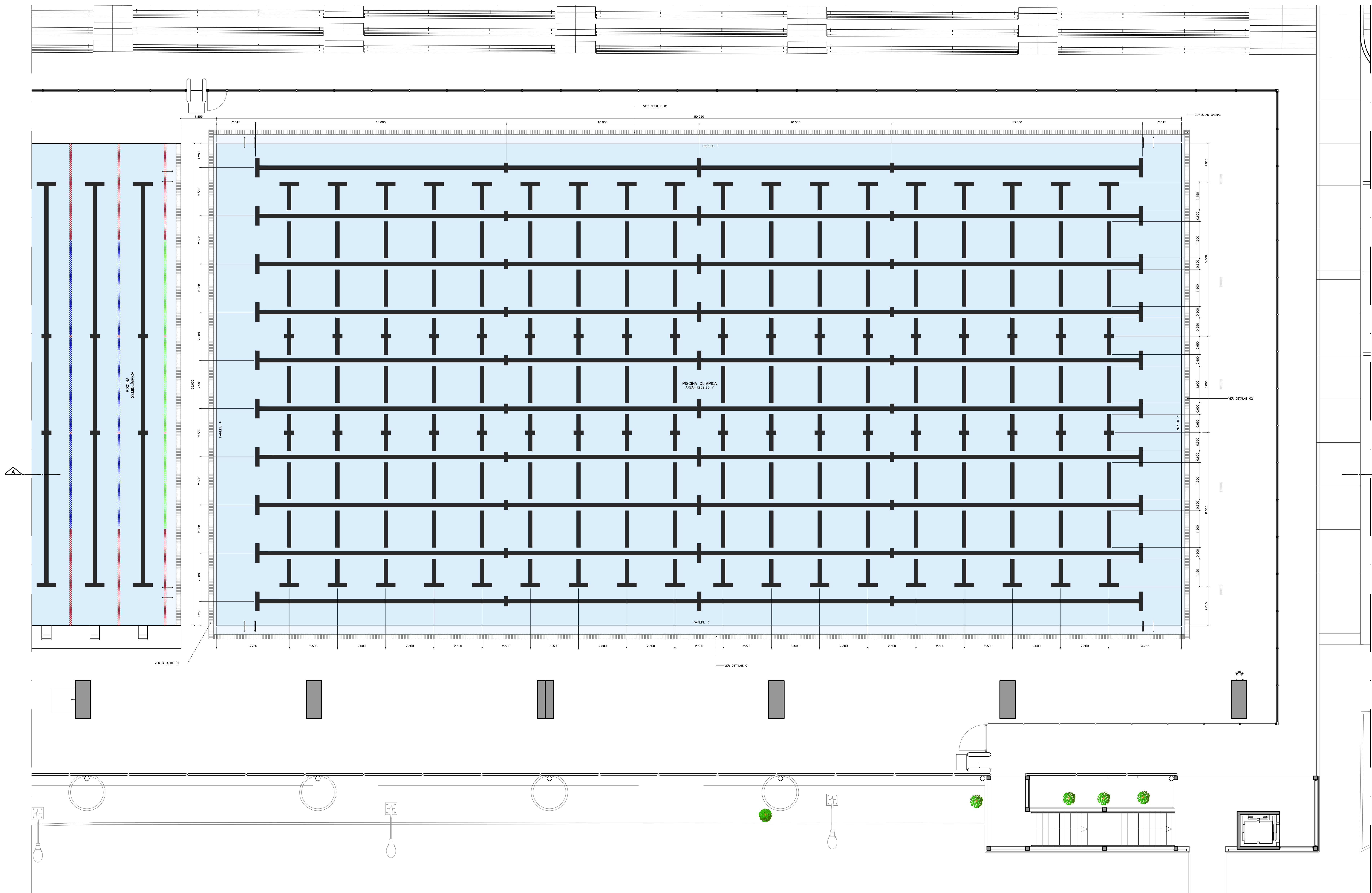
PLANTA ESC. 1:75
