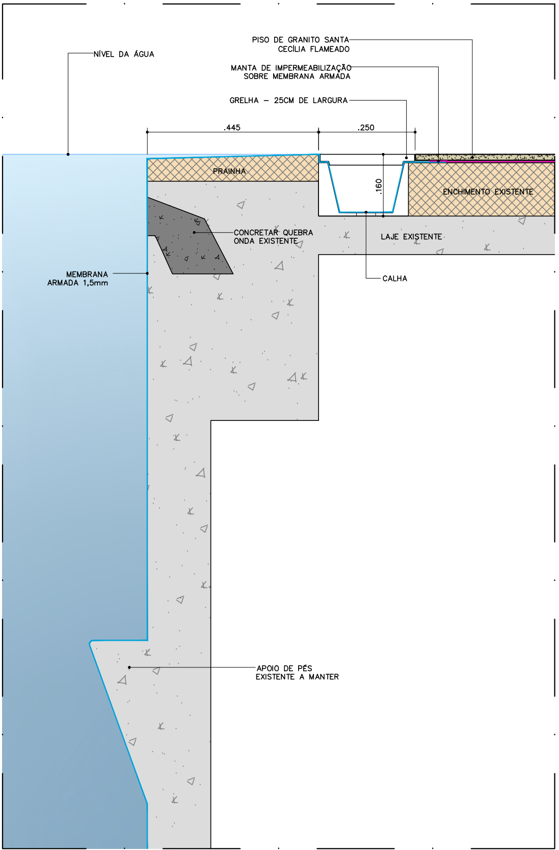
DET. 01 - CALHA PAREDES 1 E 3 ESC. 1:10
