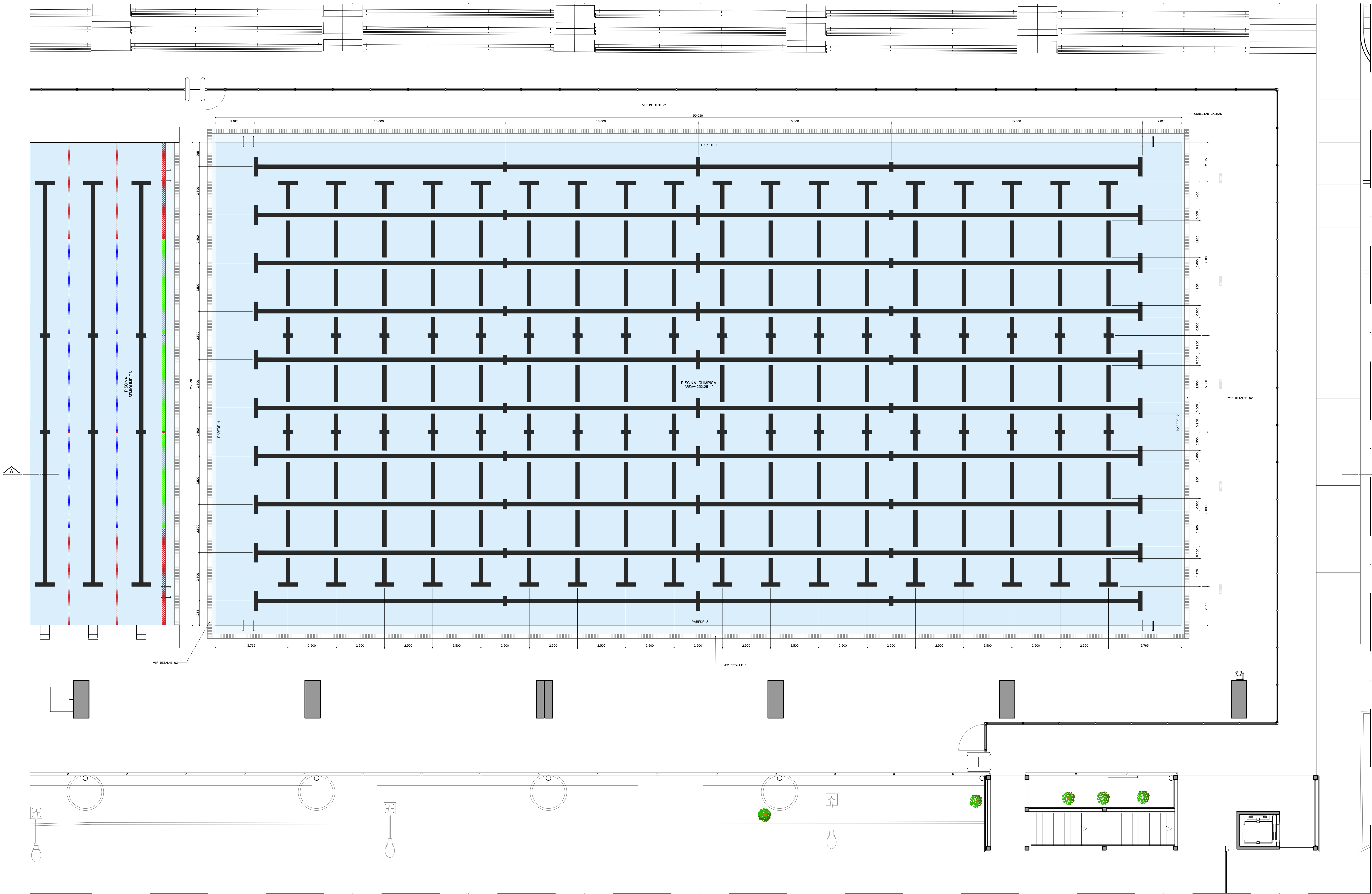
PLANTA ESC. 1:75
