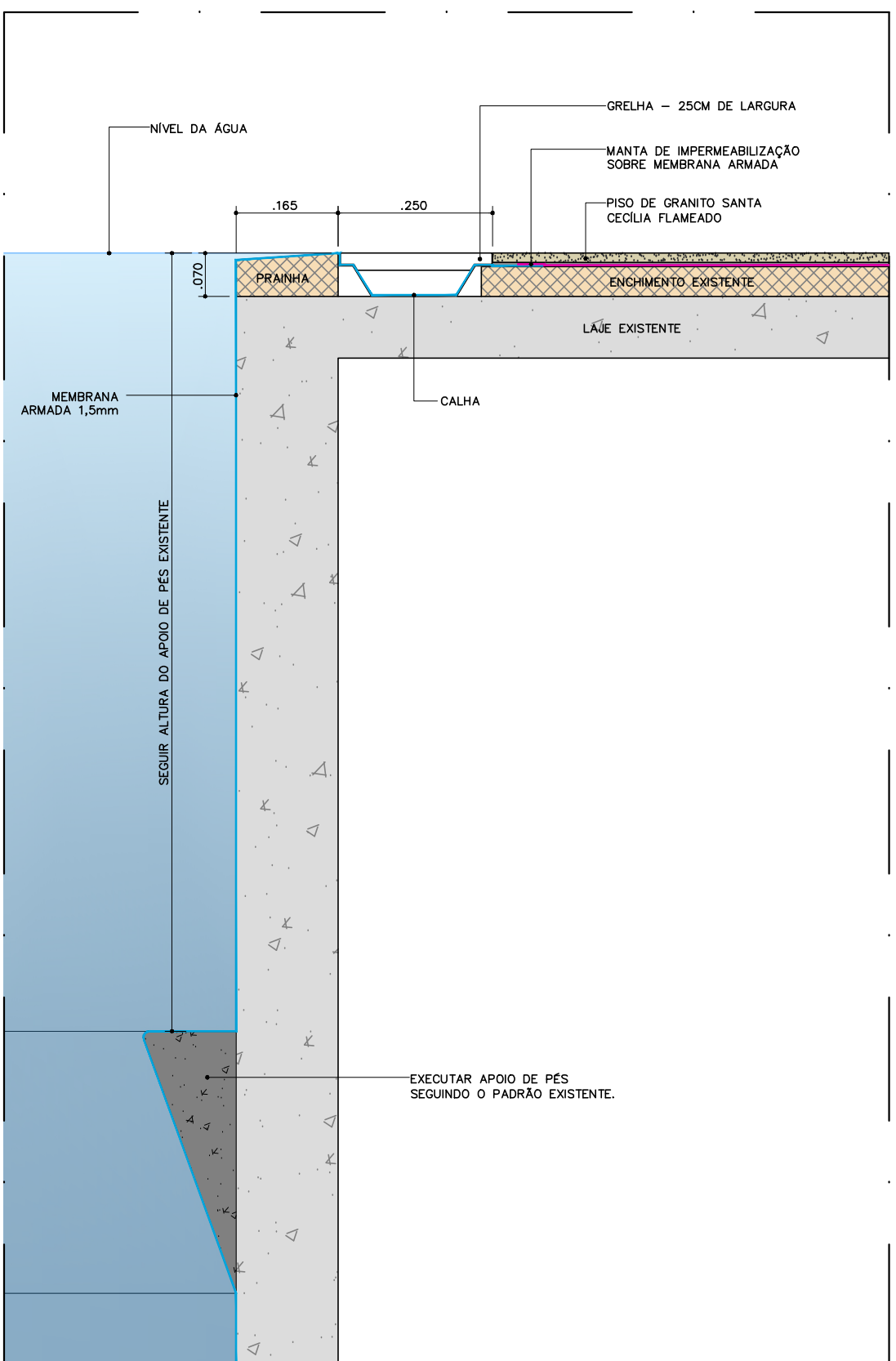
DET. 02 - CALHA PAREDES 2 E 4 ESC. 1:10
